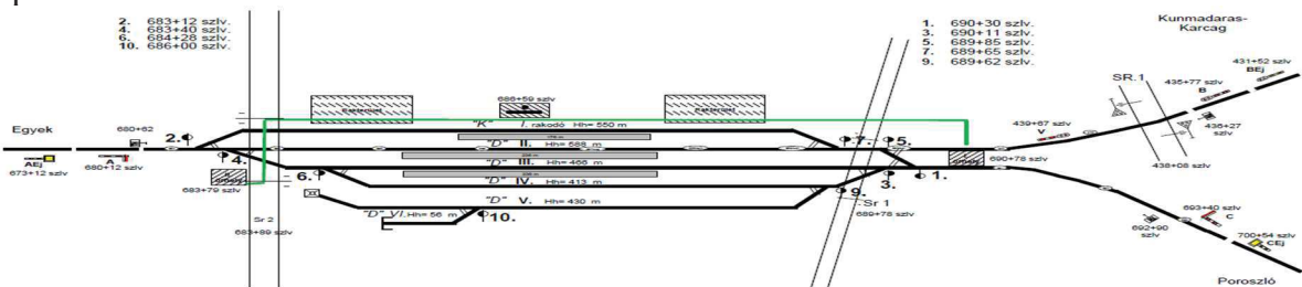
Tiszafüred állomás torzított helyszínrajza
