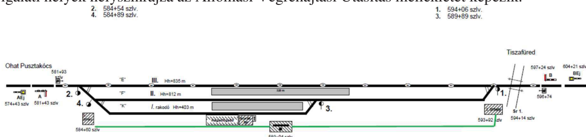
Egyek állomás torzított helyszínrajza
